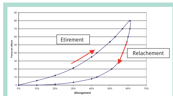
FIGURE 4 : Courbe d'hystérésis à partir d'une bande élastique.
