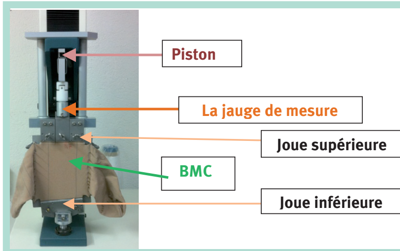
FIGURE 2 : Système IFTH France.
