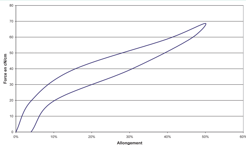
FIGURE 7 : Courbe d'hystérésis d'une bande élastique à allongement long à plat.
