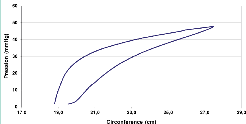
FIGURE 10 : Courbe d'un Sigvaris 504. Notez la différence de pente entre les 2 tracés.
