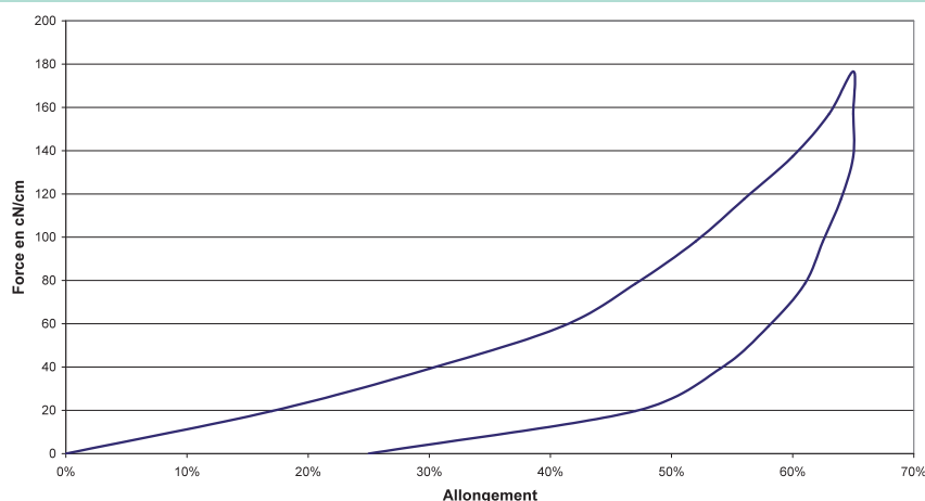
FIGURE 6 : Courbe d'hystérésis d'une bande élastique à allongement court à plat.
