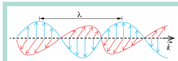
FIGURE 3 : Onde électromagnétique.
