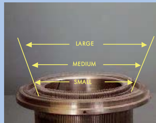
FIGURE 4 : Les 3 diamètres des métiers à tricoter
