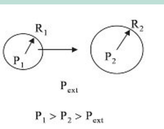
FIGURE 5 : Le mûrissement est lié à la différence de pression entre deux bulles de diamètre différent : l'air contenu dans la bulle la plus petite, diffuse vers la bulle la plus grande où la pression est plus faible selon les lois de Laplace. La mousse perd peu à peu de son homogénéité et la mousse devient beaucoup moins stable.
