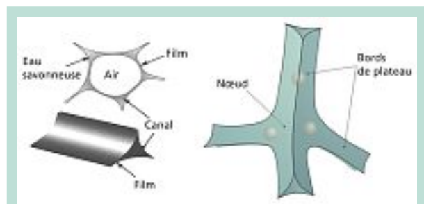
FIGURE 3 : Circulation du liquide dans le réseau de canaux séparant plusieurs bulles. Trois bords de Plateau se réunissent pour former un canal et plusieurs canaux sont réunis par un nœud.
