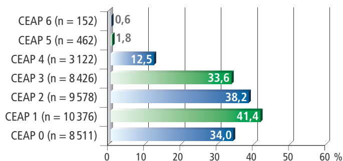
FIGURE 3 : Classement CEAP.
