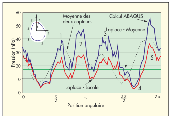
Fig. 12. – Évolution de la pression calculée par ABAQUS® et de Laplace au niveau du genou (tricot Diaphane 2) en fonction de la position angulaire
