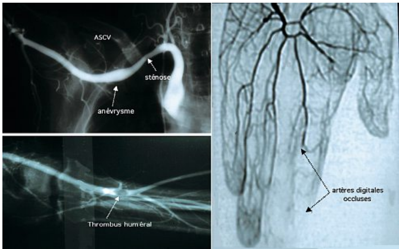
Fig. 3. – Artériographie d'un SDTB artériel ayant occasionné une sténose de l'artère sous-clavière (ASCV) avec un anévrisme post-sténotique responsable d'embols aux niveaux huméral et digital
