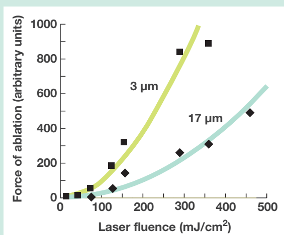
GRAPHE 5 : Effet ablatif en fonction de l'Irradiance. (Exemple).
