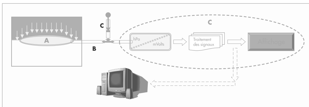
Fig. 8. ... Principe SIGaT de mesure de pression d'interface
